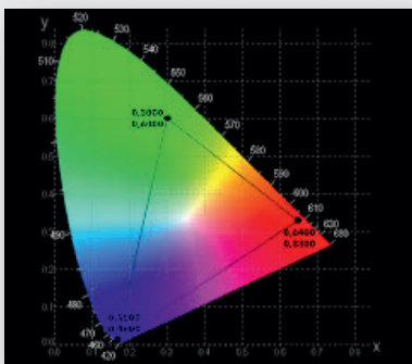
Farbtransformation im Harlequin RIP
